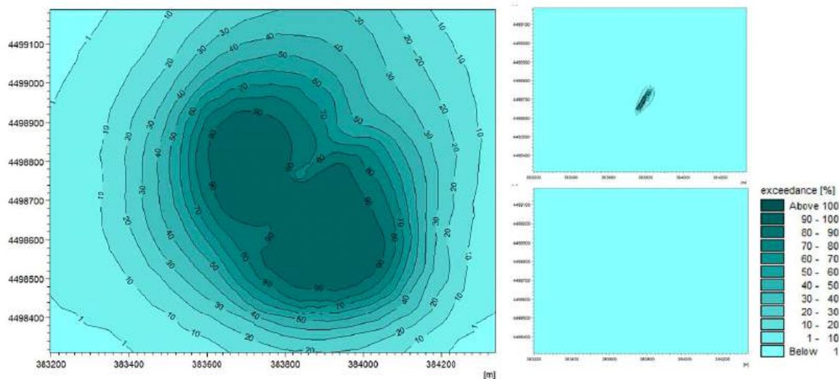
Şəkil 4-2 Duzluluq fərquində 1 PSU həddinin aşılma müddəti
